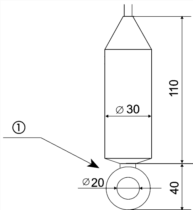
PulsFox® PMG 20 - 62/63 Verankerungsöse
