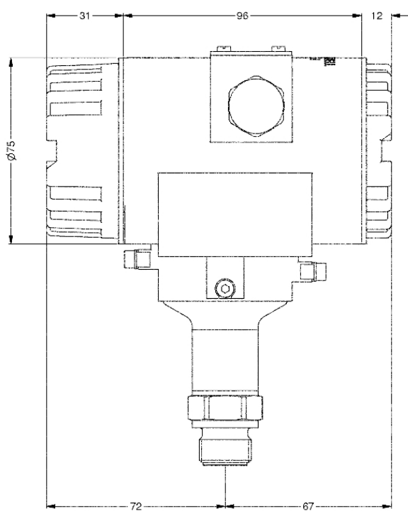
Masse (mm)
