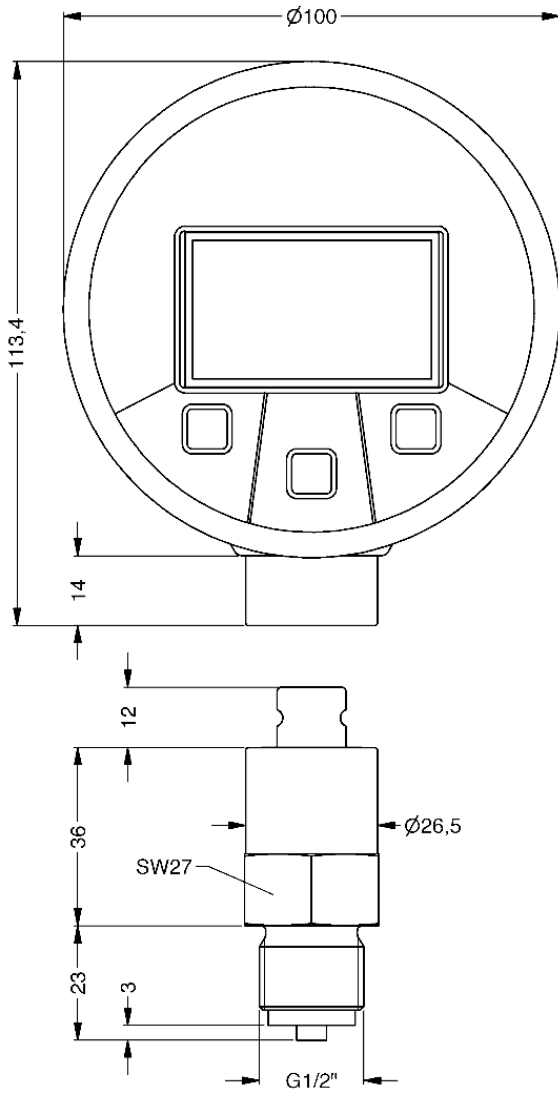
Masse (mm)
