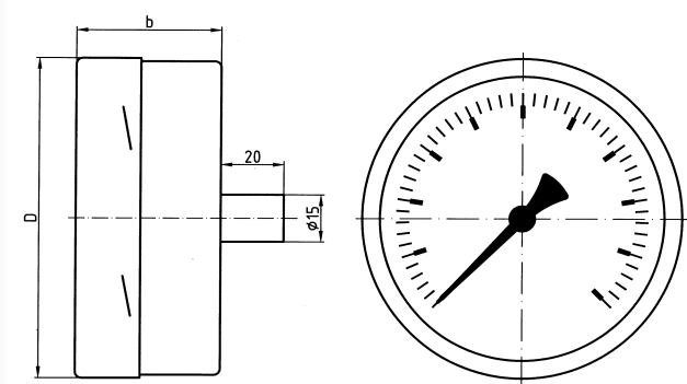
Anschluss axial
