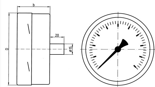
Maße (mm)
