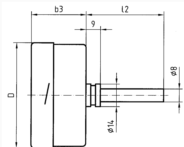
Anschluss axial, glatt
