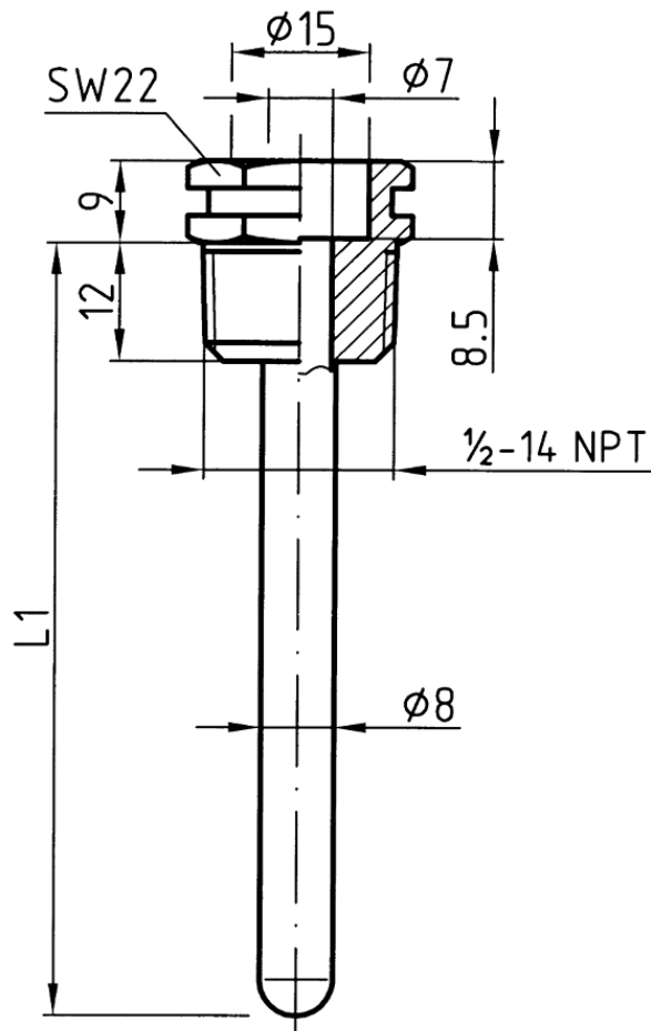
Tauchhülse ½" 7 x 8 mm
