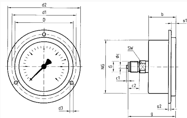
Masse (mm)
