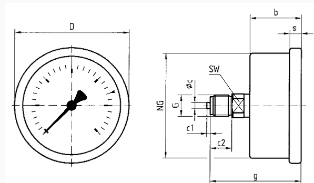
NG 50/63 – Anschluss axial
