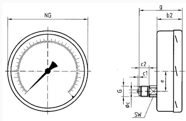
Masse (mm)
