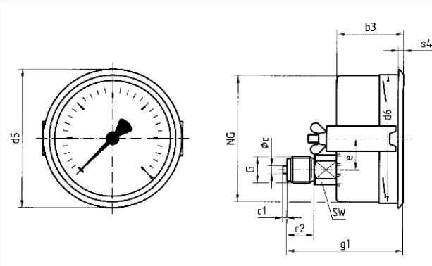
Anschluss axial exzentrisch, 3-Kantfrontring mit Bügelbefestigung
