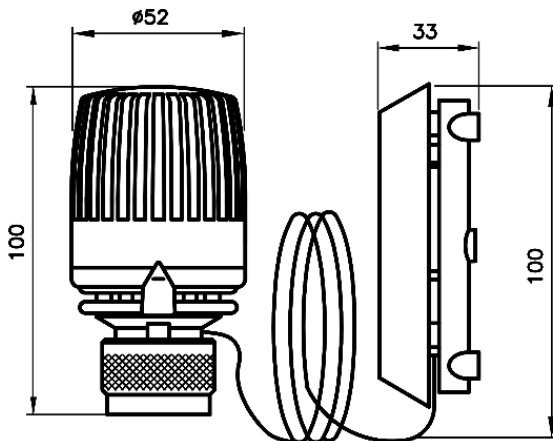
Thermostat-Regelkopf 323 KD mit Fernfühler, Danfoss-Klemmanschluss
