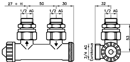
Vario THK M, Eck – Ausführung G½ Aussengewinde
