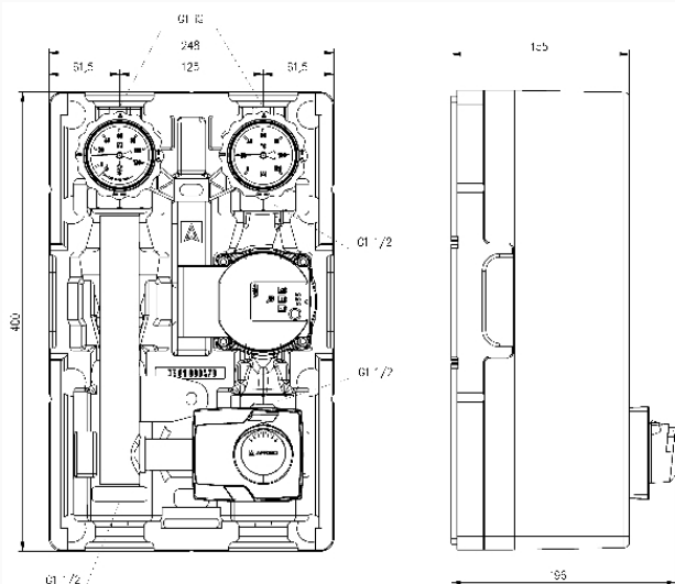
PrimoTherm® 180-2 mit Wilo-Pumpe
