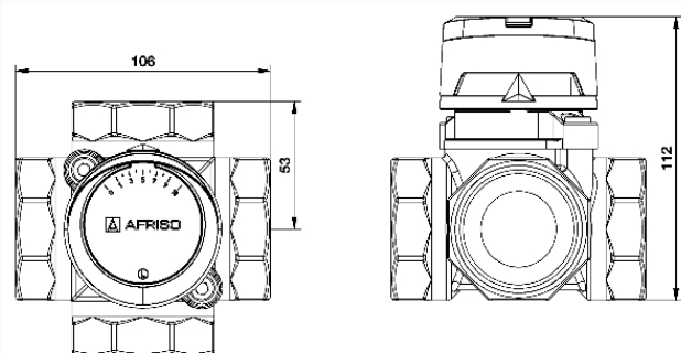
4-Wege-Mischventil DN 40
