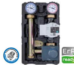
Heizungspumpengruppe PrimoTherm® K 180-2 DN 25 KVS Vario als kurze Aus- führung, mit einstellbarem Kvs-Wert von 2,5 bis 12 m³/h
