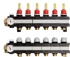
Kunststoff-Heizkreisverteiler ProCalida® MC 1 für Heizen & Kühlen
